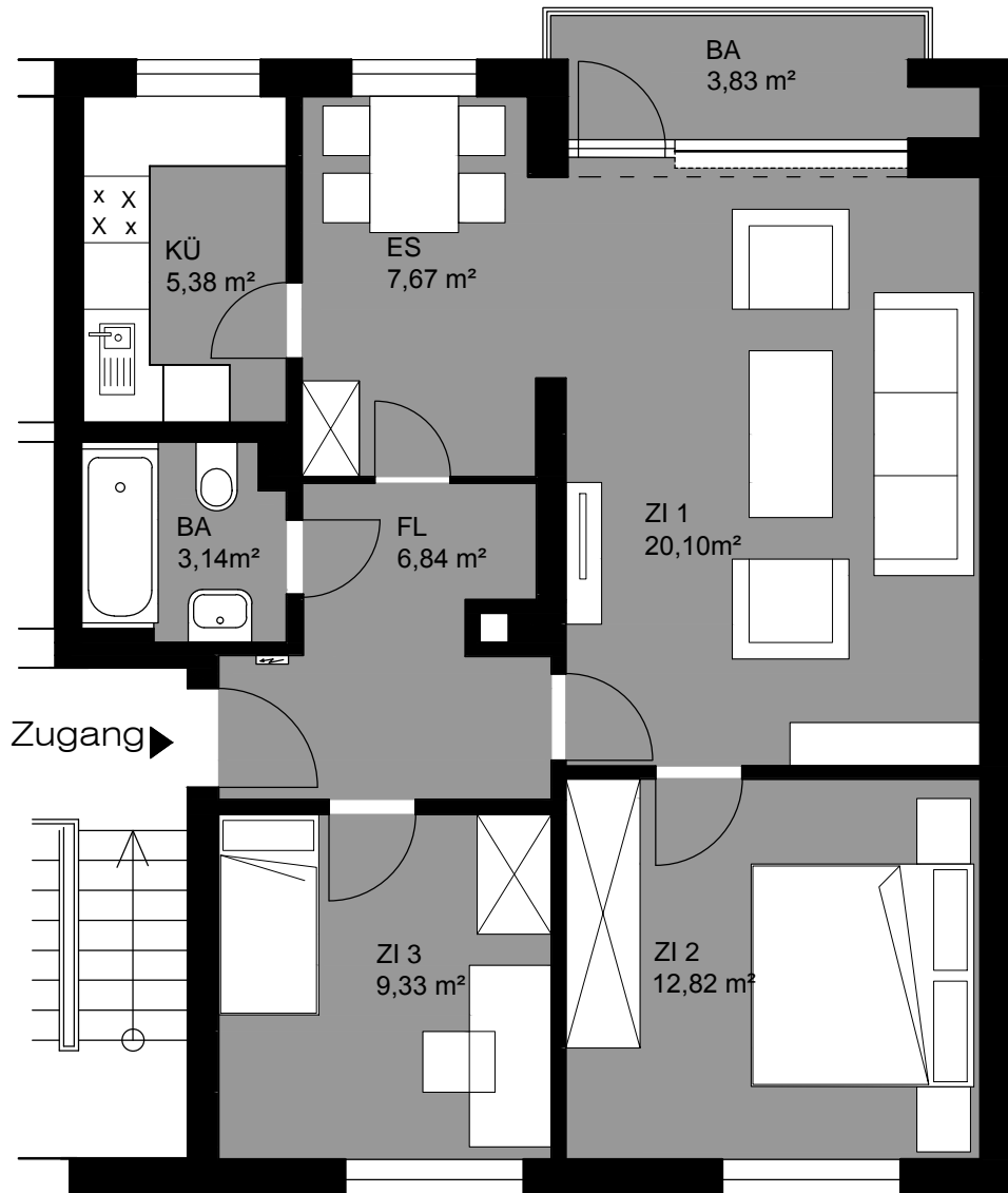
OBERGESCHOSS rechts
