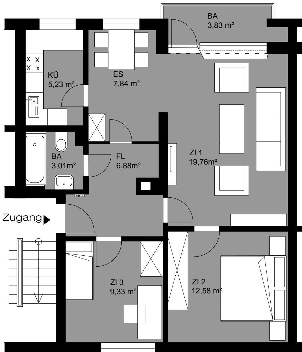
OBERGESCHOSS rechts
